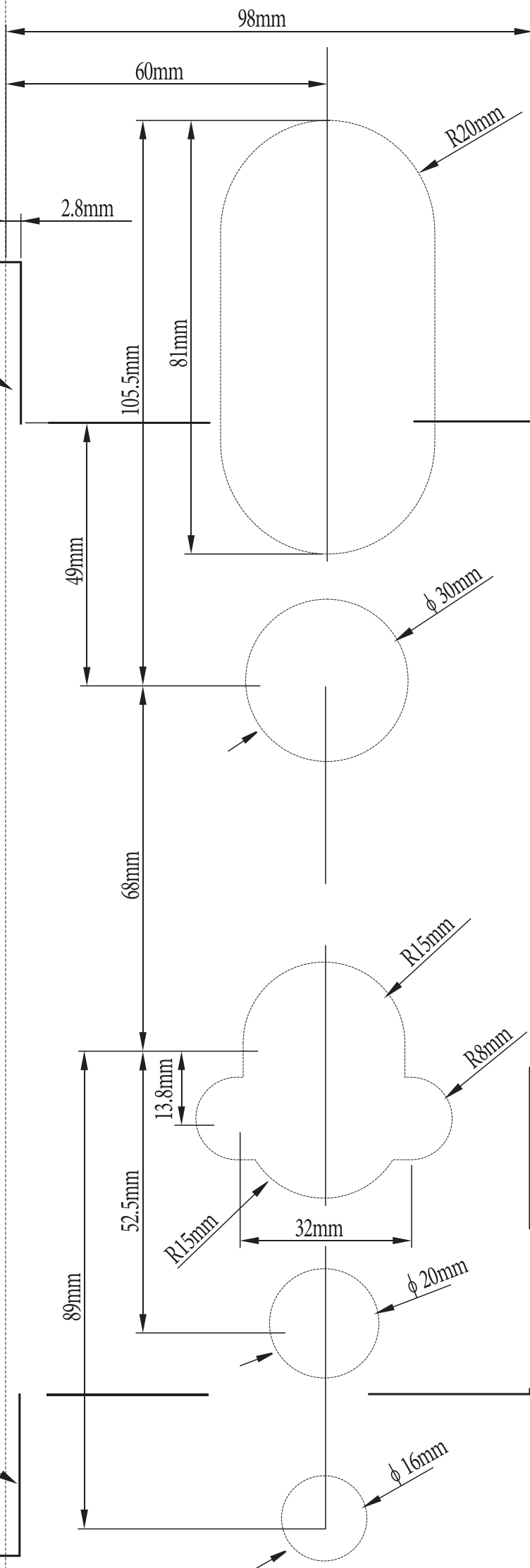
6068锁体开孔图 1 : 1
